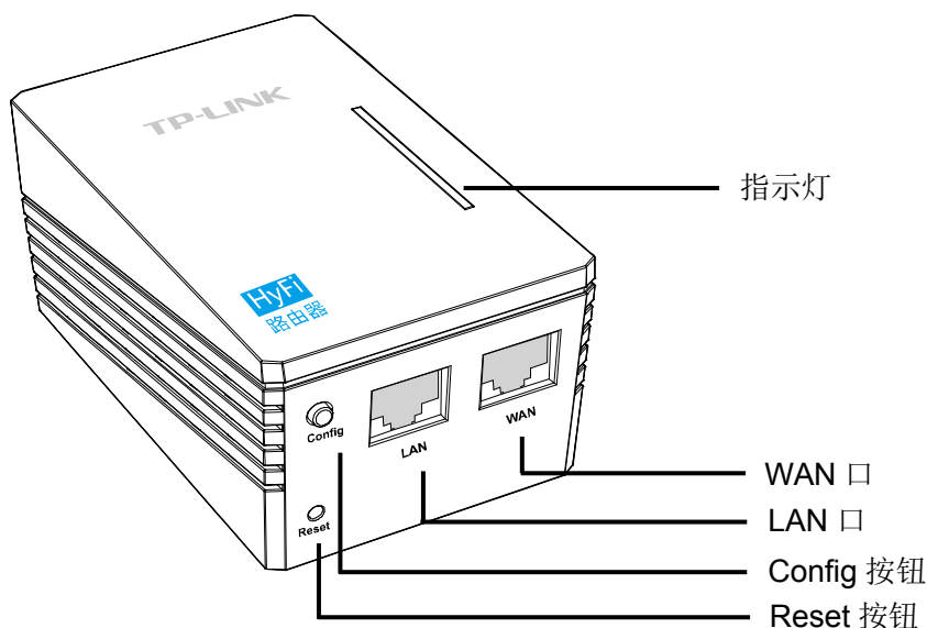
图 3-1 TL-H29R 示意图
