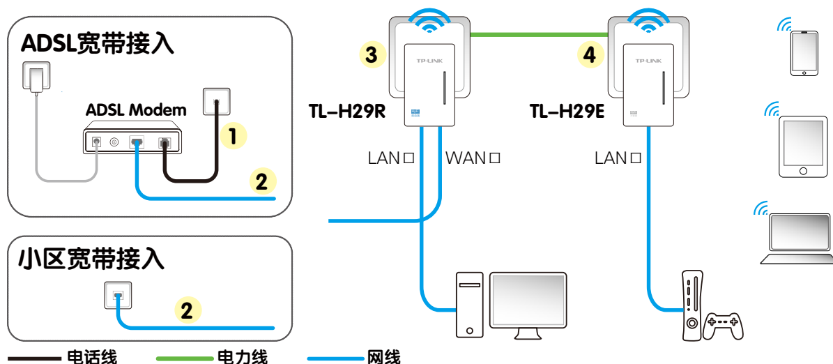
图 4-1 TL-H29R/TL-H29E 硬件安装示意图
